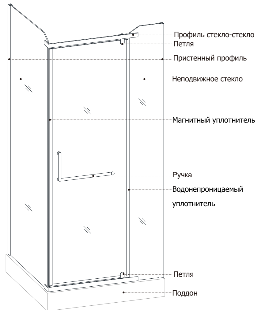
Общий вид душевого угла
